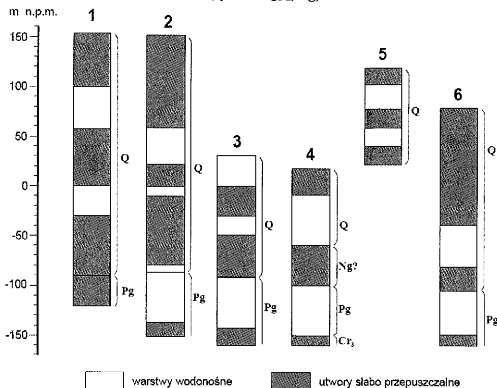
Rysunek 8. Profil JCWPd-19 (symbol Q 1-2 , Pg)
