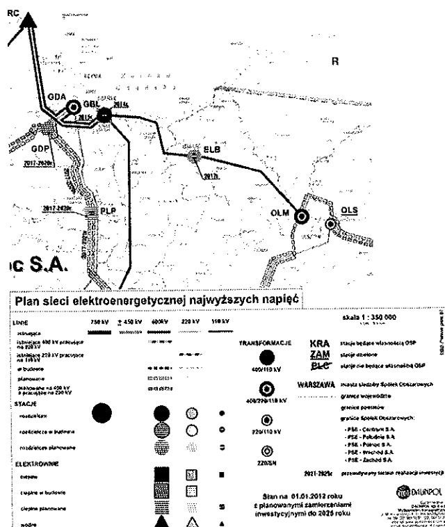
Rysunek 25. Przebieg linii 400 kV przez teren powiatu elbląskiego
